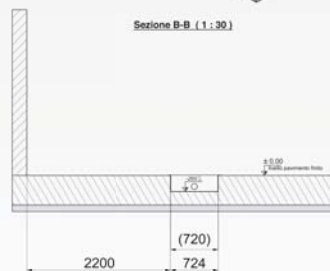
Sezione B-B (1:30)
